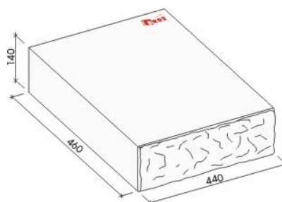
Brož Muráno® schodišťový blok
