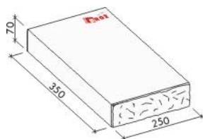
Brož Muráno® 7 / 35 stříška
