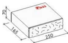
Brož Muráno® 7 / 16,5 základní kámen
