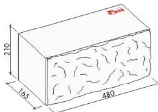
Brož Muráno® 21 / 16,5 základní kámen
