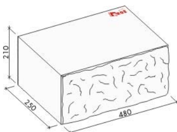
Brož Muráno® 21 / 25 základní kámen
