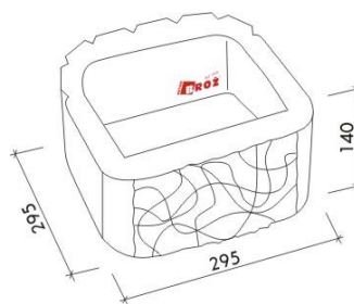
Svahová tvarovka štípaná
