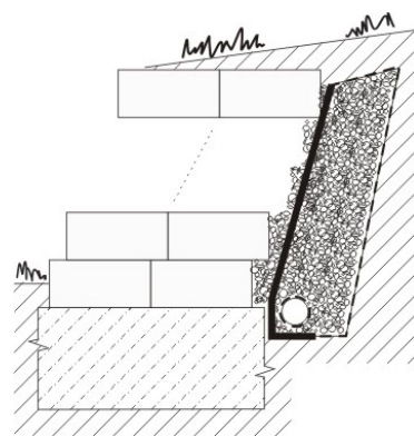
Obrázek č.2: Kládkování betonových tvarovek ve dvou řadách za sebou
