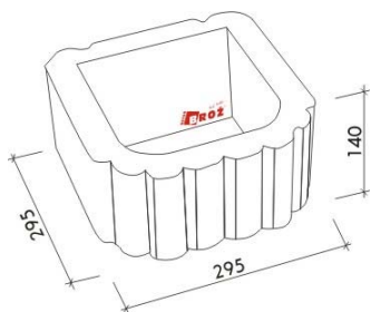
Svahová tvarovka hladká
