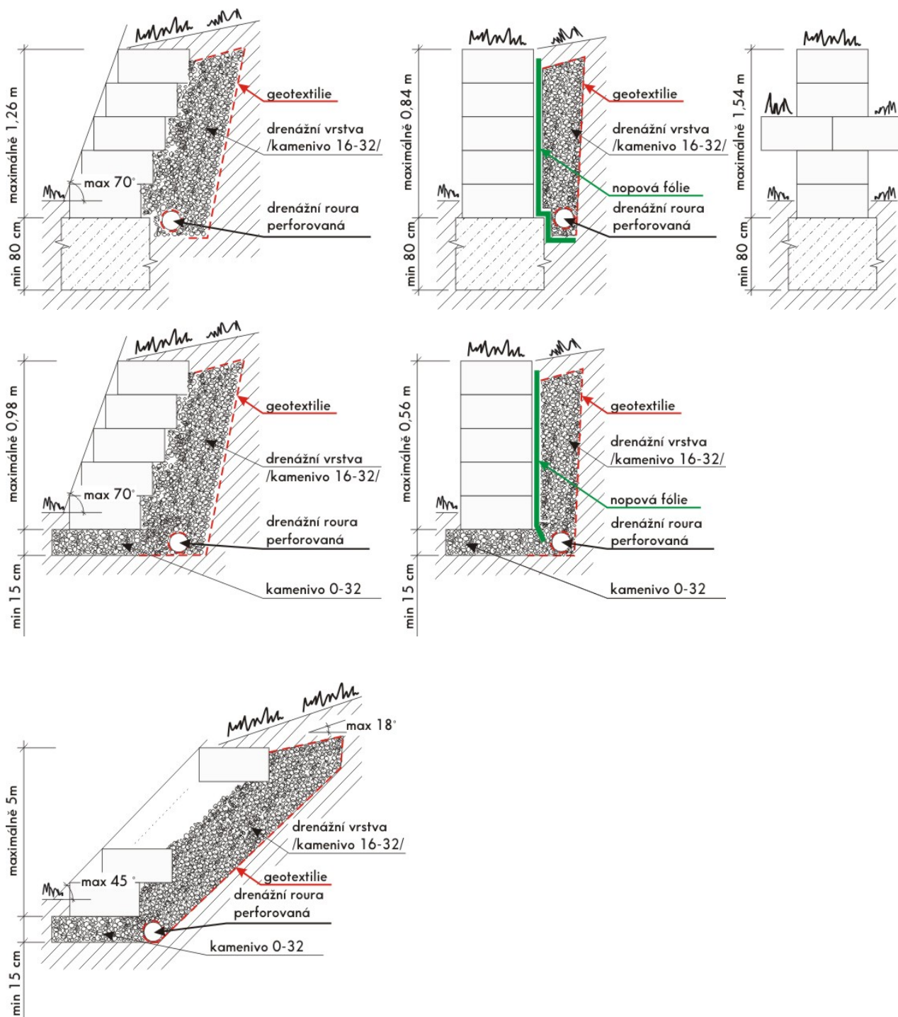
Obrázek č.3: Zásady výstavby samostatně stojících a opěrných konstrukcí
