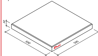
Dlaždice 50 / 50 / 5,5 (povrch BROŽ Standard)
