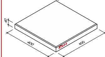
Dlaždice 40 / 40 / 5 (povrch BROŽ Standard)
