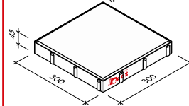
Dlaždice 40 / 40 / 4 (povrch BROŽ Praktik)
