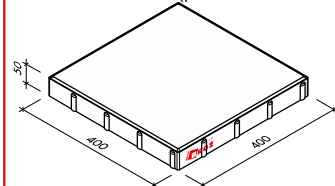
Dlaždice 50 / 50 / 5, Mocca (povrch BROŽ Praktik)
